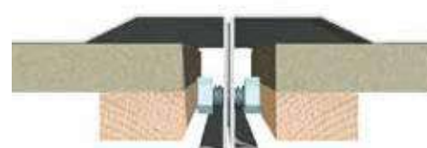
Koppelverbinding met bouten met WK4 randafwerking
