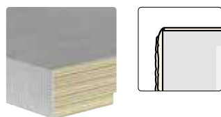
2 mm PPFR-rand 50 en 62 mm hoog met facet
